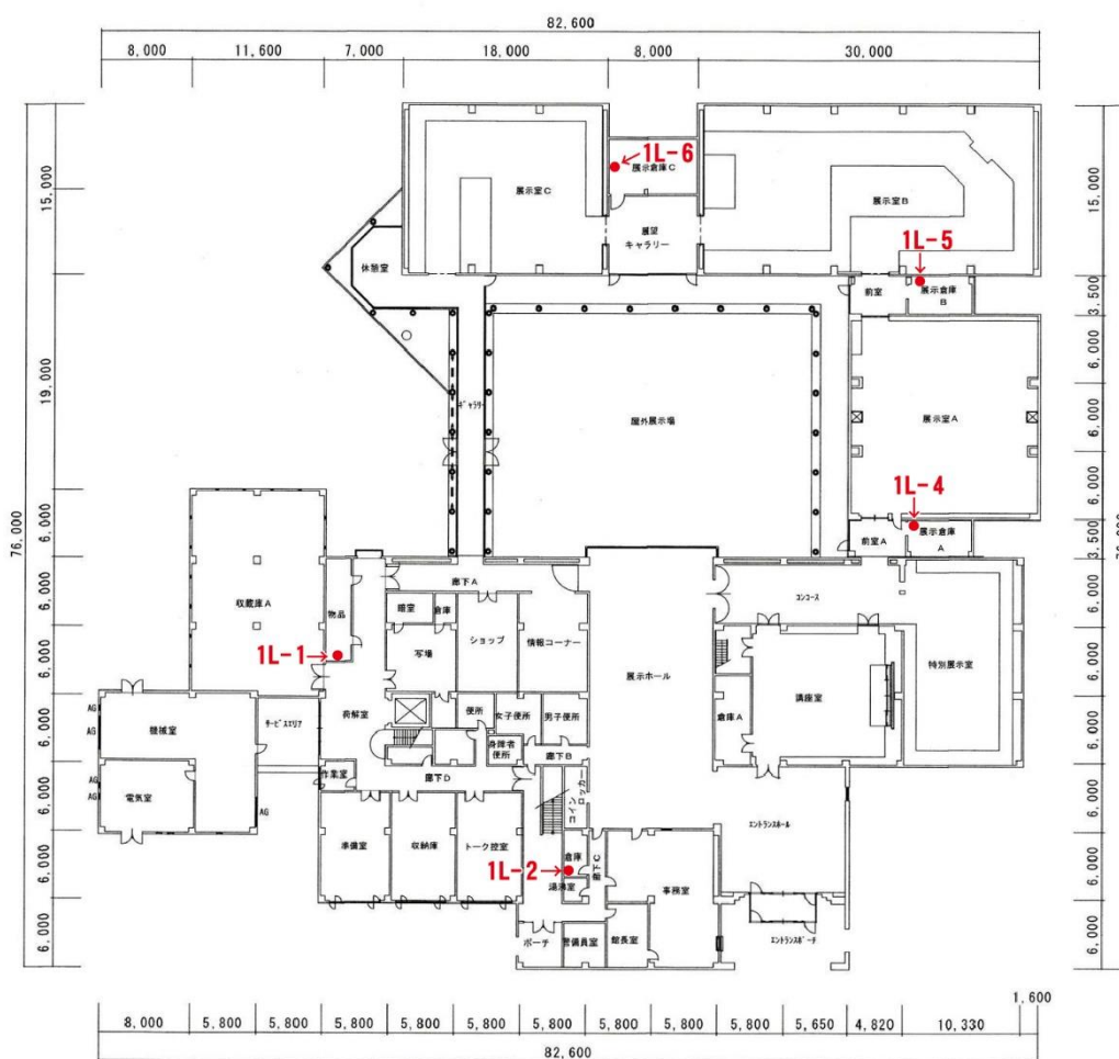
分電盤配置図
